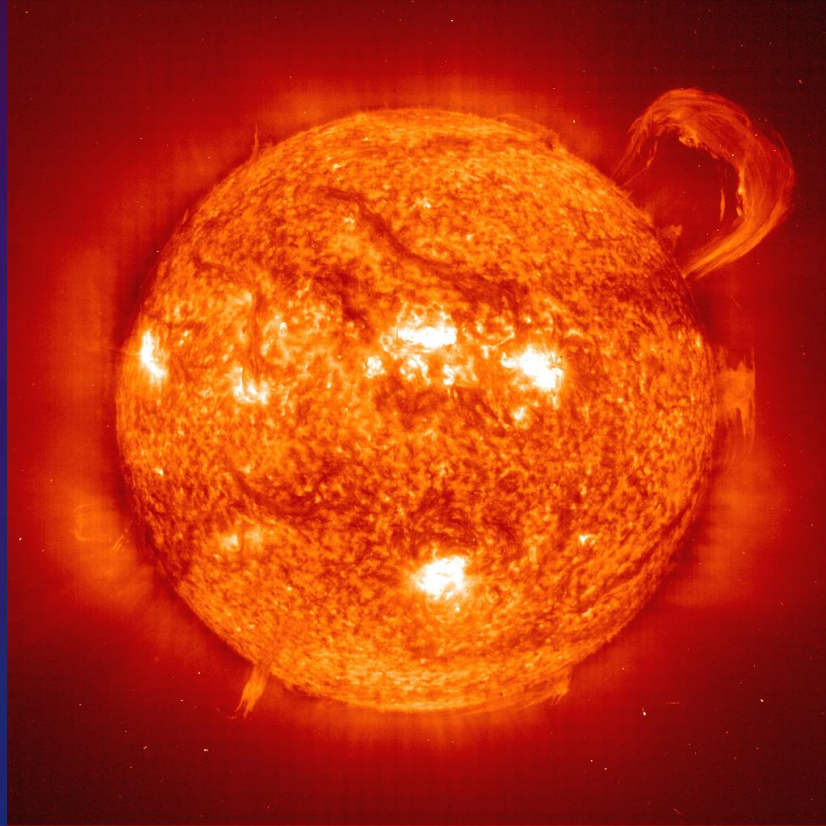
Sol
