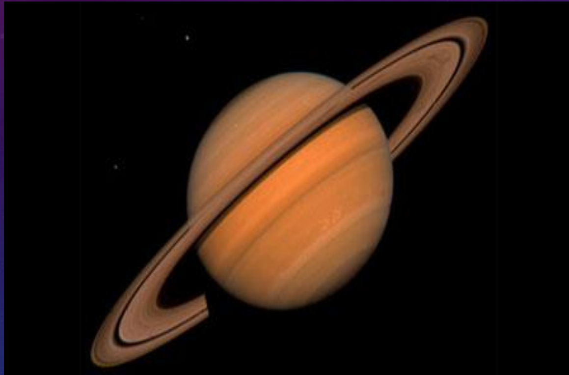
Saturno
